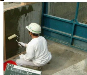
〈塗布中〉
